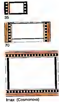
Фотоматеріали Кіноплівка (широка стрічка використовується у деяких системах панорамного кіно) 35 мм (нормальна стрічка) 70 мм (широка стрічка) Imax (стрічка проходить через камеру горизонтально)
